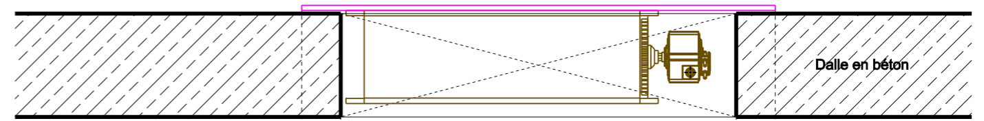
Coupe A-A
